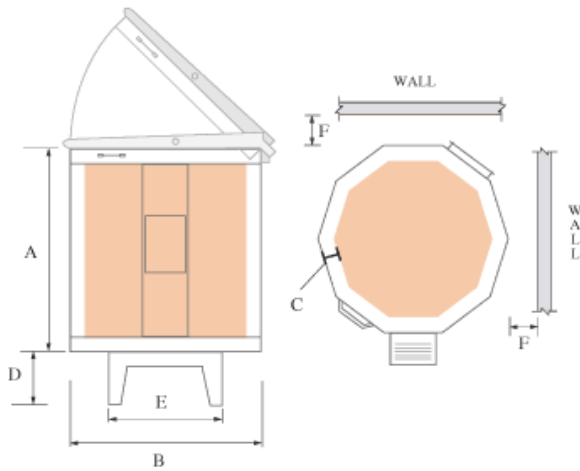
DIMENSIONS
