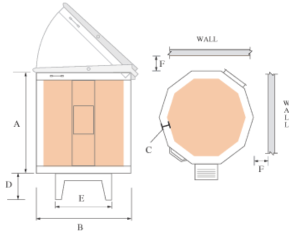
DIMENSIONS
