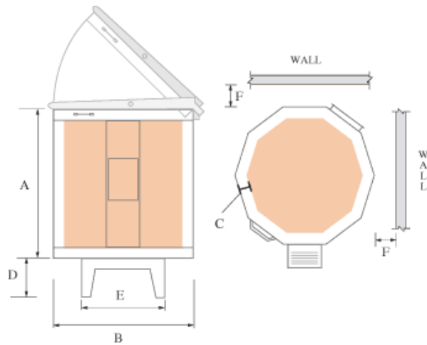
DIMENSIONS
